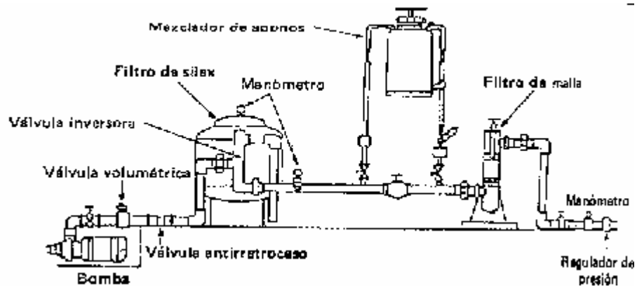
Figura 2. Cabezal de riego tipo
