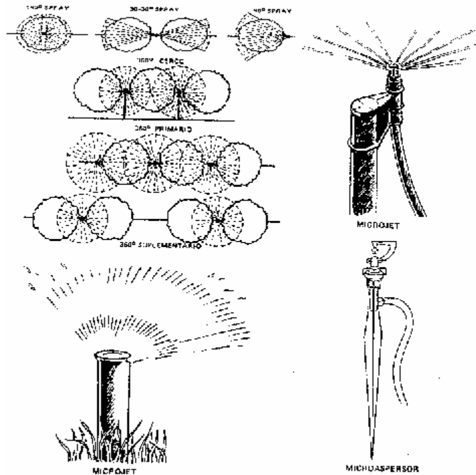
Figura 11. Características de microjet y microaspersores.
