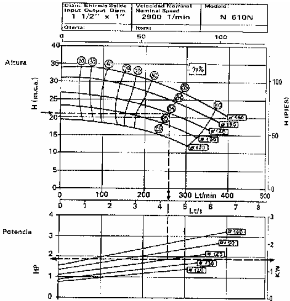
Figura 3. Curva característica de una bomba tipo.
