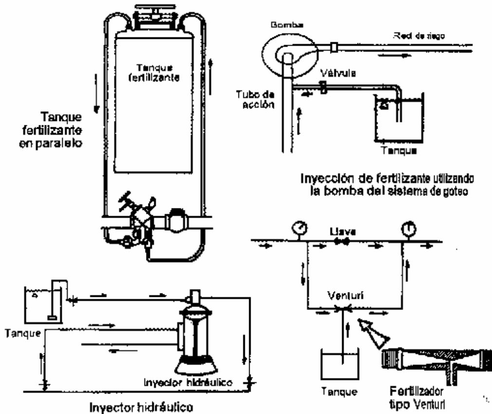
Figura 7. Diferentes sistemas de aplicación de fertilizantes en riego por goteo
