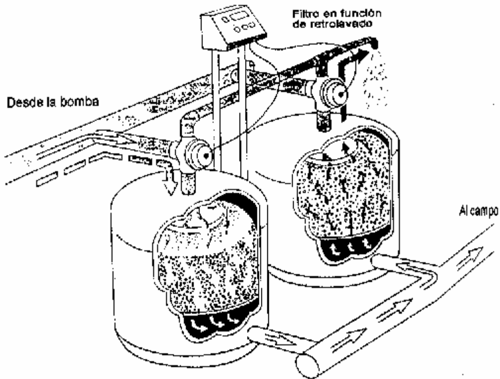
Figura 5. Retrolavado en filtros de arena y programador de riego.
