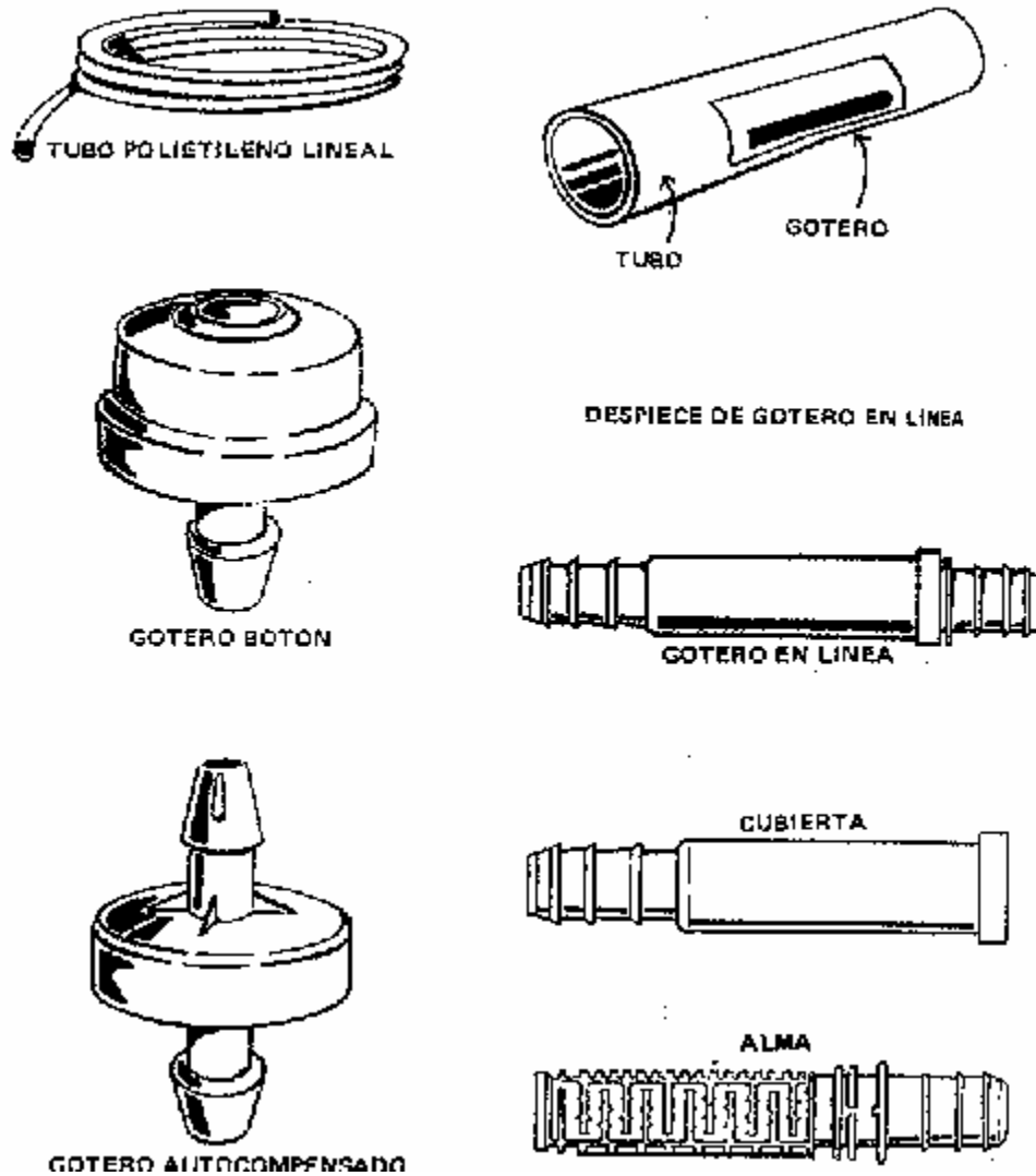
Figura 9. Diferentes tipos de goteros en Chile
